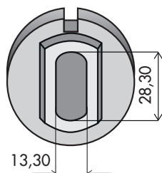
PUNZÓN OVALADO Ref. P8
