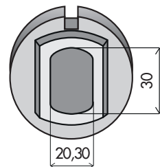
PUNZÓN OVALADO Ref. P7
