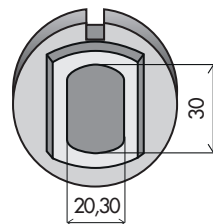
PUNZÓN OVALADO Ref. P7
